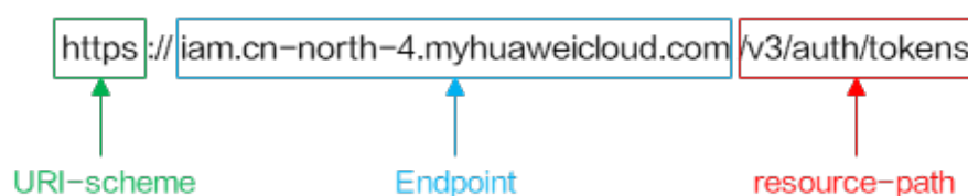
图 3-1 URI 示意图
