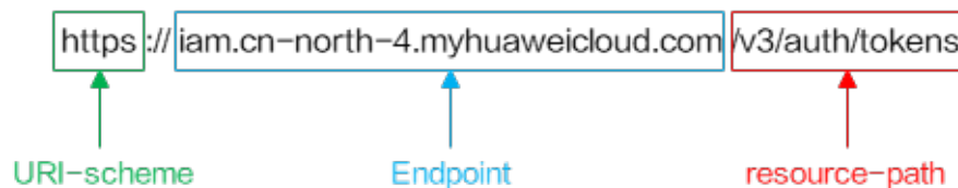
图 2-1 URI 示意图
